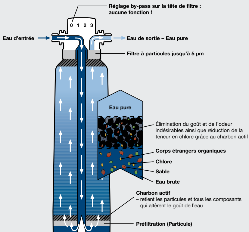
Structure d'une cartouche filtrante besttaste
